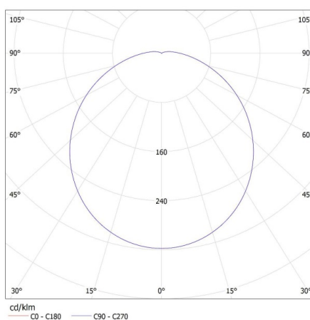
MILED0 (kat 30412) DUNO LED 24W-WW-O / Krzywa rozsyłu światła (biegunowo)
