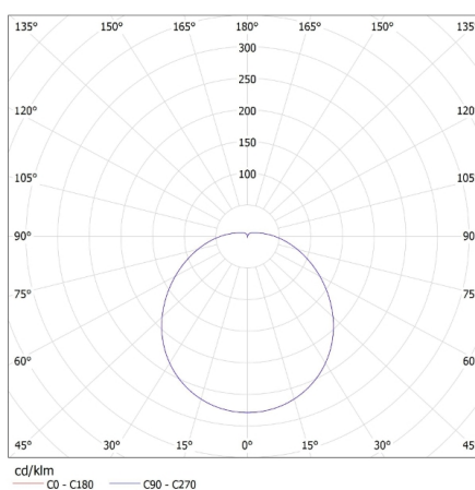
MILEDO (kat 31098) CORSO LED N 24-NW / LDC (Polar)
