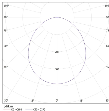
KANLUX S.A. (kat 22825) TOMI LED7W GU10-NW / LDC (Polar)
