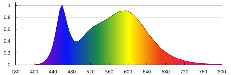
KANLUX S.A. (kat 22825) TOMI LED7W GU10-NW / LDC (Polar)
