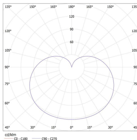
KANLUX S.A. (kat 27302) IQ-LED G45E14 5,5W-CW / LDC (Polar)
