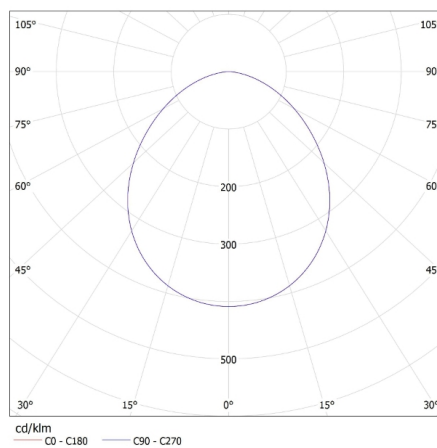
MILED0 (kat 31015) GU10 LED N 4W-NW / LDC (Polar)
