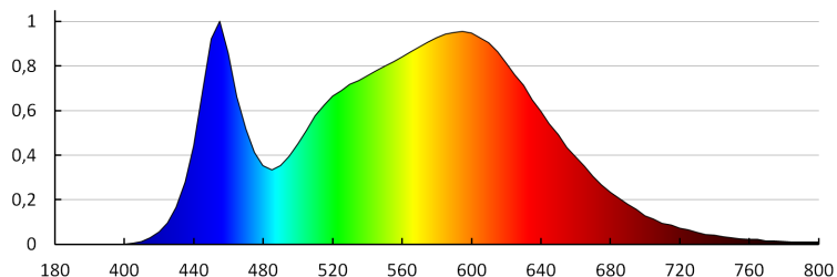
MILED0 (kat 31015) GU10 LED N 4W-NW / LDC (Polar)
