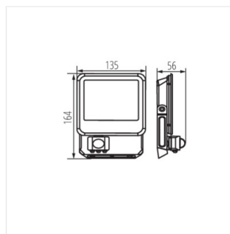
IQ-LED FL-10W-NW-SE
