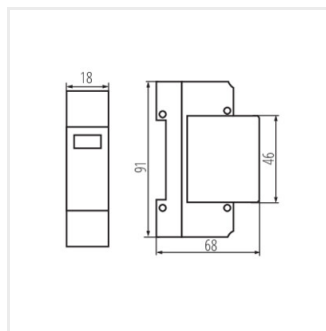
KSPD-T2 275/40 1P
