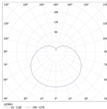
KANLUX S.A. (kat 22571) LUNI PRO E27 LED-WW / Krzywa rozsyłu światła (biegunowo)
