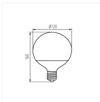
LUNI PRO E27, LUNI MAX E27
