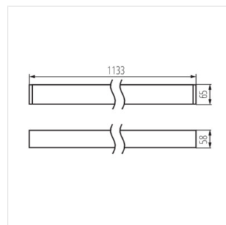
AL 23W-840-MPR-W-NT
