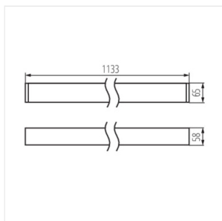
AL 23W-840-MPR-B-NT
