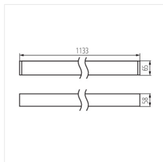
AL 23W-840-MPR-SR-NT
