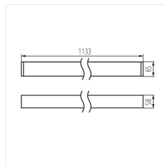
AL 23W-840-MAT-SR-NT
