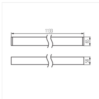
AL 23W-830-MAT-B-NT
