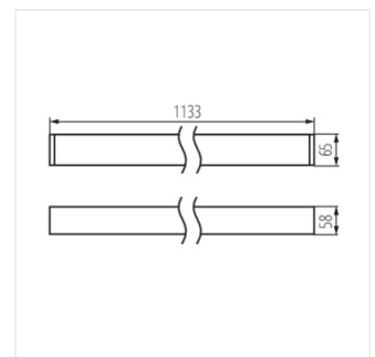
AL 23W-840-RST-B-NT
