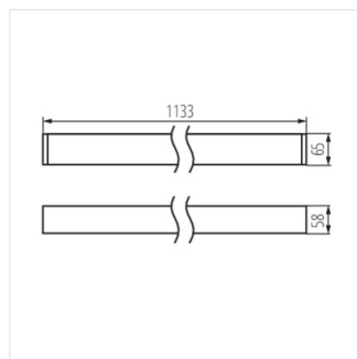
AL 23W-840-MAT-B-NT
