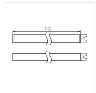
AL 23W-840-MAT-W-NT
