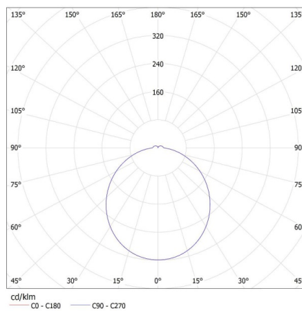
KANLUX S.A. (kat 26442) VARSO LED 18W-WW-L / Krzywa rozsyłu światła (biegunowo)
