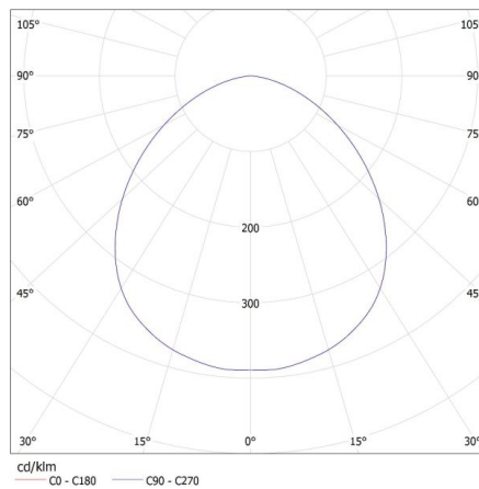
KANLUX S.A. (kat 22191) PAX TL-60LED / Krzywa rozsytu światła (biegunowo)
