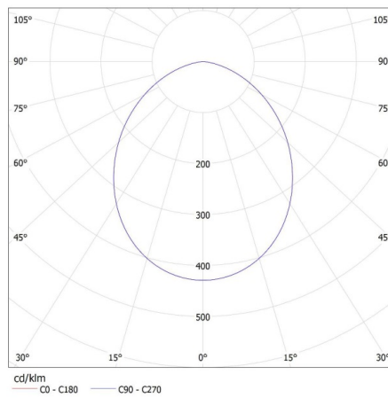
KANLUX S.A. (kat 25511) TIBERI LED SMD 36W / Krzywa rozsyłu światła (biegunowo)
